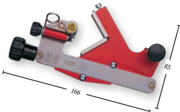
Dụng cụ lột vỏ cáp FBS - 1722 1
